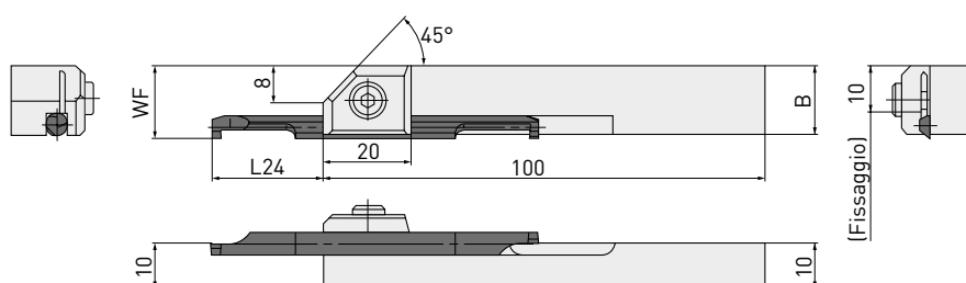
Tipo CG (la barra per alesatura si inserisce in uno stelo)
