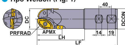
● Tipo Weldon (Fig. 1)
