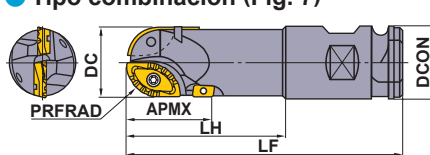
● Tipo combinación (Fig. 7)
