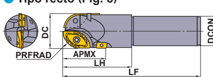
● Tipo recto (Fig. 8)
