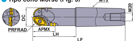
● Tipo cono Morse (Fig. 5)
